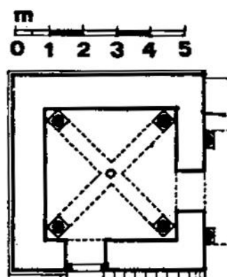
Zadar, samostan benediktinki, prostorija u prvom katu zvonika, tlocrt (Jeran-Pohl 1975, 91)
