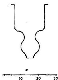
profilacija rebra sakristije zagrebačke katedral, prema Z. Horvat 1992, 75 (lijevo) i prema Weiss 1859 (desno)
