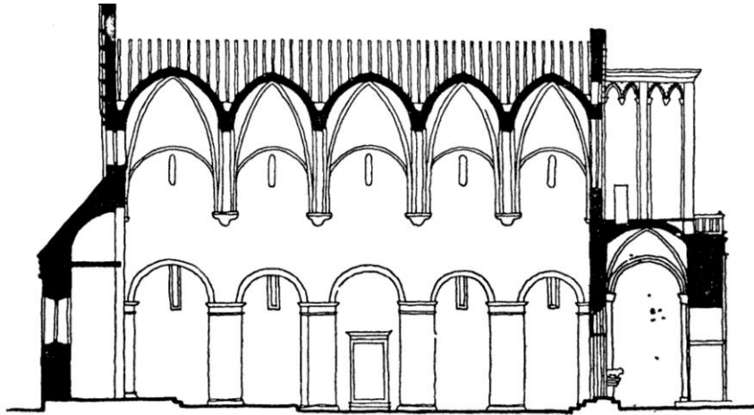
Trogirska katedrala, uzdužni presjek (prema: A. Deroko; Subotić, 1963, 57)
