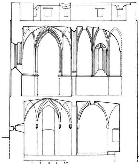
Brinje, dvorska kapela Presvetog Trojstva, presjek kroz brod kapele i bočnu južnu kapelu (Horvat, Z. 1985, 57, sl. 23)
