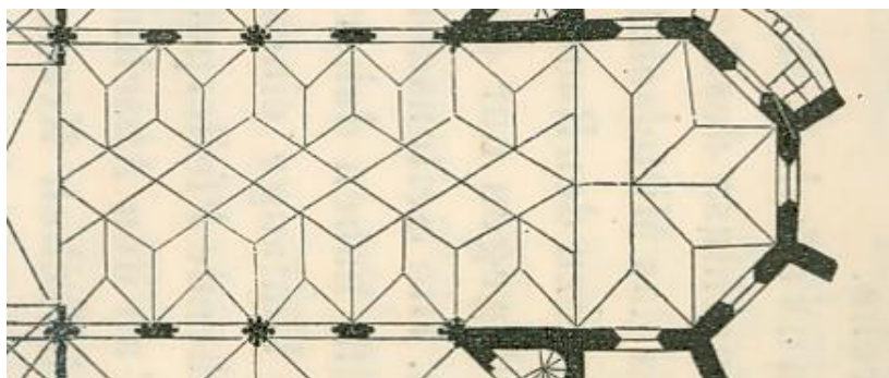
Zagrebačka katedrala, glavni brod svetišta, stanje prije regotizacije, tlocrt (Weiss 1859, 233, sl. 1)
