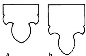
Rebra s bademastim zaključkom i zaliscima a. Čazma, crkva sv. Marije Magdalene b. Medvedgrad, kapela sv. Filipa i Jakova (Horvat, Z. 1992, 74, sl. 80a, b)
