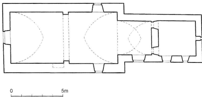
Zaglav, franjevačka crkva, tlocrt (Marković 2008, 130)
