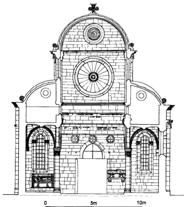
Šibenska katedrala, poprečni presjek kroz uzdužne brodove (Zavod za fotogrametriju) Radovi IPU 3-6, 1982, 261, sl. 5.
