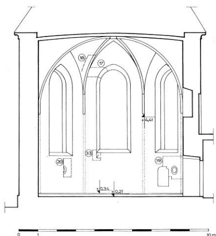
Nedelišće, Presveto Trojstvo, župna crkva, poprečni presjek (Srša, 1993, 10)
