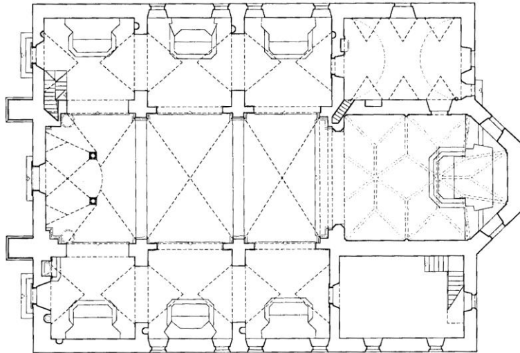
Pazin, župna crkva sv. Nikole, tlocrt (Marković, V. 2004, sl. 70)
