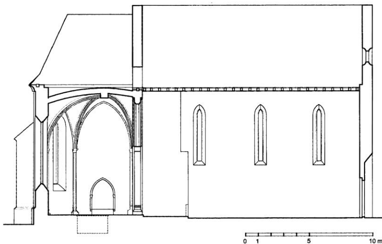
Požega, crkva sv. Lovre. Idejna rekonstrukcija prve gotičke faze, uzdužni presjek (Srša 2005, 25)
