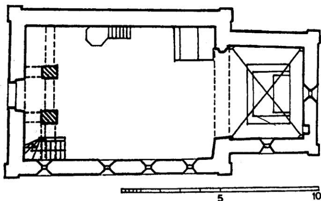
Kapela sv. Petra i Pavla u Novom Mjestu kod Zeline, tlocrt (Horvat, Z. 2004, 35) profilacije rebara (Horvat Z, 1977, 6)
