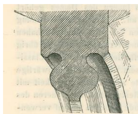
profilacija rebra sakristije zagrebačke katedral, prema Z. Horvat 1992, 75 (lijevo) i prema Weiss 1859 (desno)
