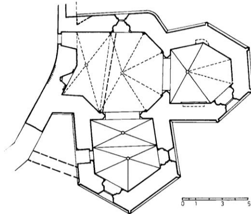
Brinje, dvorska kapela Presvetog Trojstva, tlocrt (Horvat, Z. 1985, 53, sl. 14)
