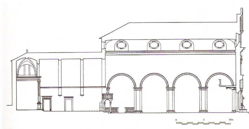
Hvarska katedrala, presjek (snimak: Tenšek – Stepinac)
