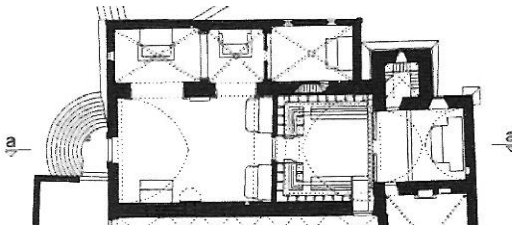
Hvar, franjevačka crkva Gospe od Milosti, tlocrt (Fisković 2010, 82)
