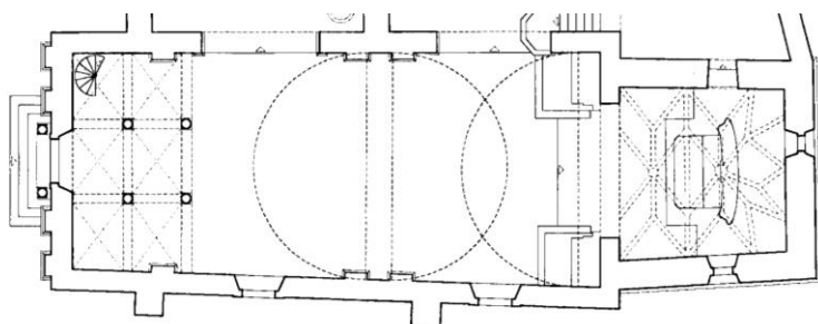
Lovran, župna crkva sv. Jurja, tlocrt (Marković, V. 2004)
