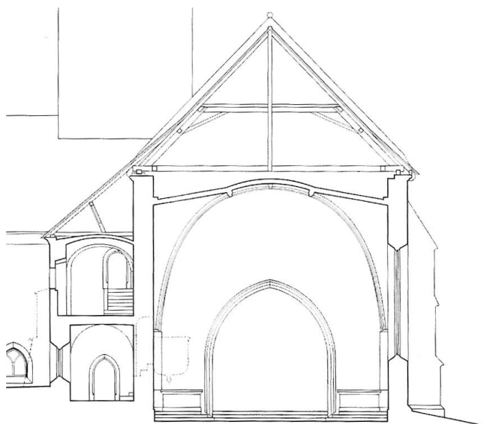
Remetinec, Sv. Marija, poprečni presjek kroz brod (Vukičević-Samaržija 1993, 199, sl. 193)
