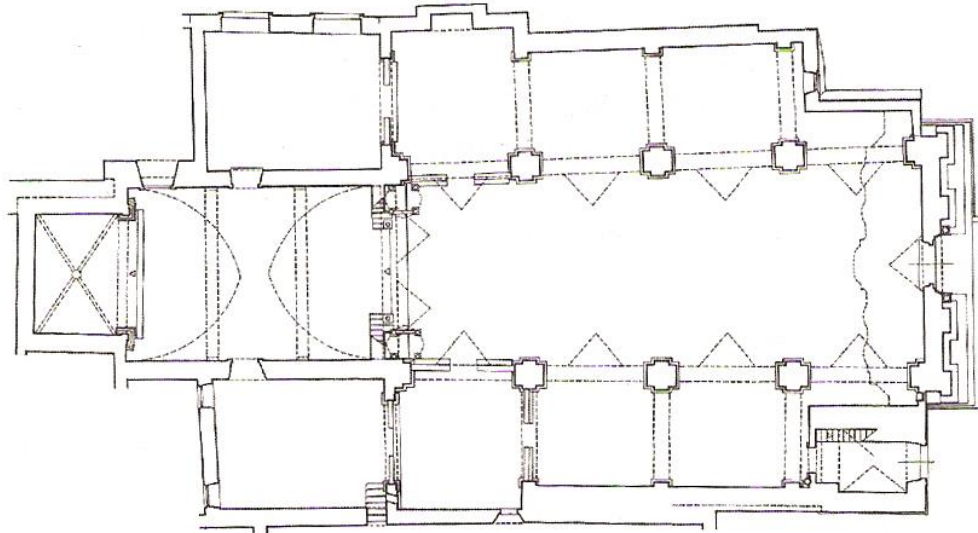
Hvarska katedrala, tlocrt (snimak: Tenšek – Stepinac)
