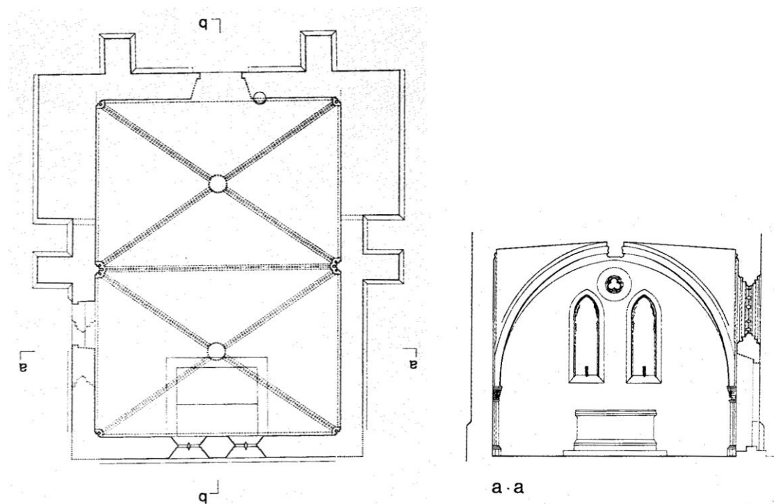
Biskupska kapela sv. Stjepana Prvomučenika, tlocrt i poprečni presjek prema jugu (prema Deanović 1988, 28)
