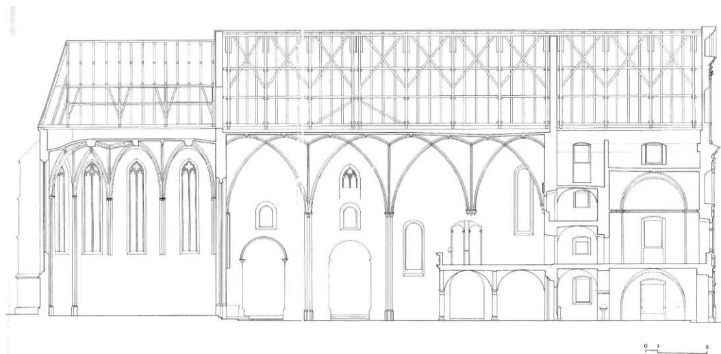
Lepoglava, crkva Bezgrešnog Začeca Blažene Djevice Marije, uzdužni presjek (Vukičević-Samaržija 1993, 168-169, sl. 163)
