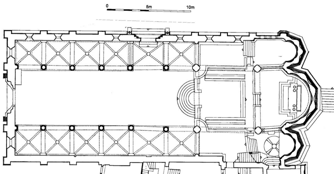
Šibenska katedrala, tlocrt (Institut za povijest umjetnosti) Radovi IPU, 3-6, 1982, 259, sl. 2
