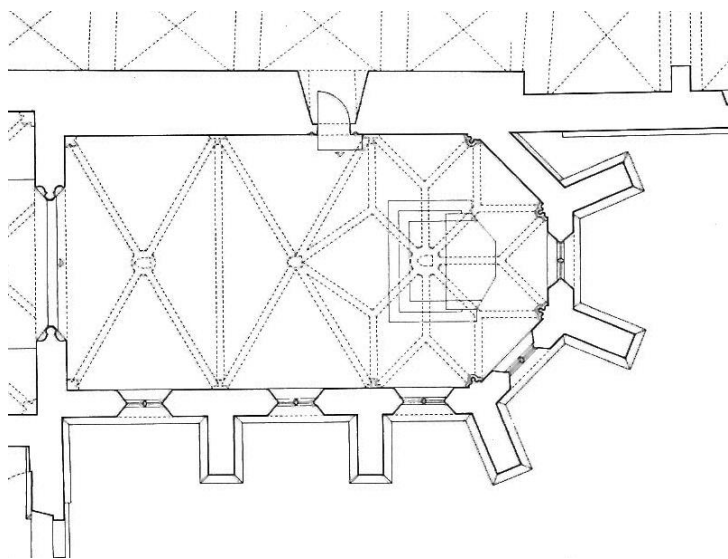
Lepoglava, crkva Bezgrešnog Začeca Blažene Djevice Marije, svetište, tlocrt (Vukičević-Samaržija 1993, 167, sl. 162)
