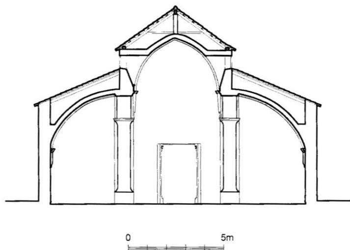
Jelsa, župna crkva sv. Fabijana i Sebastijana, poprečni presjek (Marković, 2008, 133)
