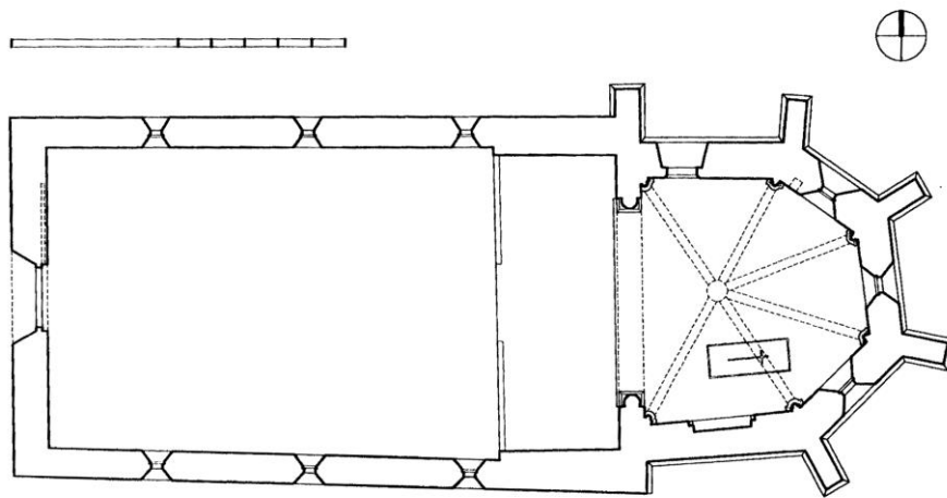
Požega, crkva sv. Lovre. Rekonstrukcija tlocrta prve gotičke faze (Srša 2005, 24)
