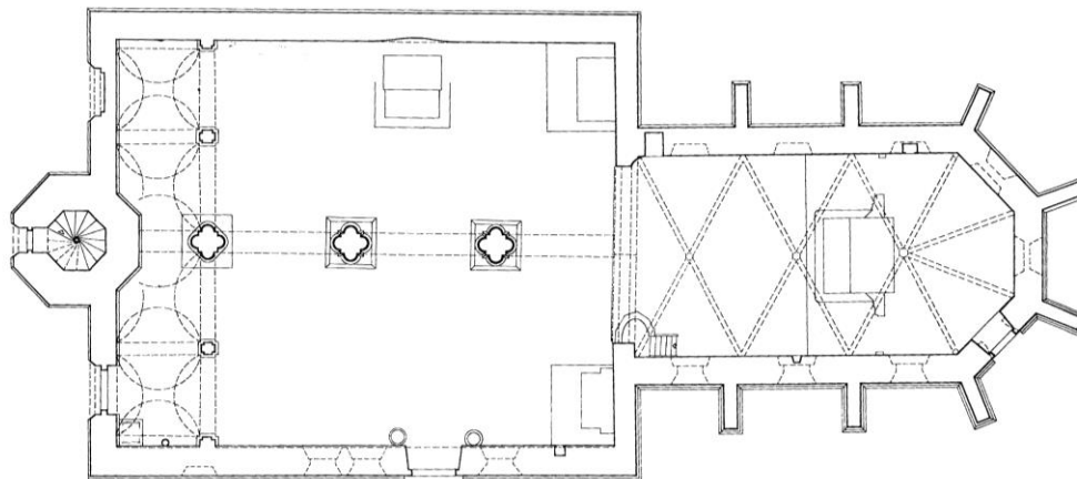
Glogovnica, župna crkva Uznesenja Blažene djevice Marije, tlocrt (Badurina 1993, 309)
