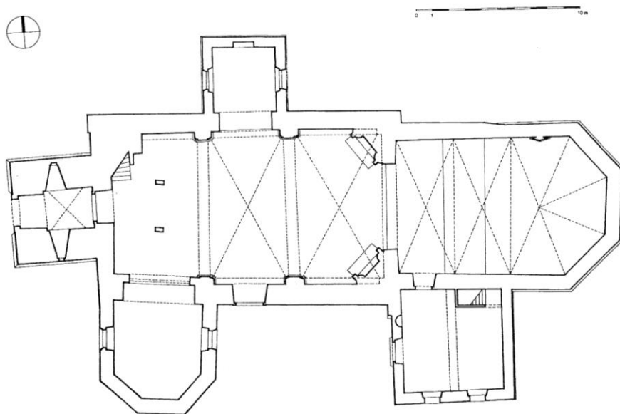
Nedelišće, Presveto Trojstvo, župna crkva, tlocrt (Srša, 1993, 7)
