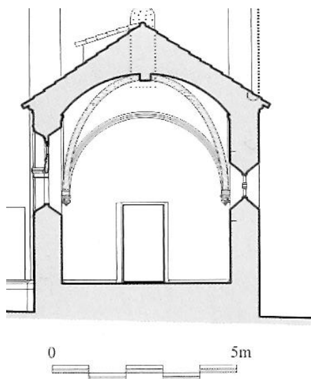
Kapela sv. Jeronima, rekonstrukcija izvornog stanja, presjek prema jugu (Tenšek & Valjato Vrus; izvor: Zelić 2007, 69)
