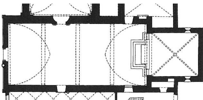
Badija - Otok kraj Korčule, franjevačka crkva, tlocrt (Fisković 2010, 91)
