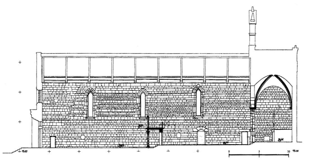
Pula, franjevačka crkva sv. Franje, uzdužni presjek (Krizmanić 2001, 86, sl. 18)
