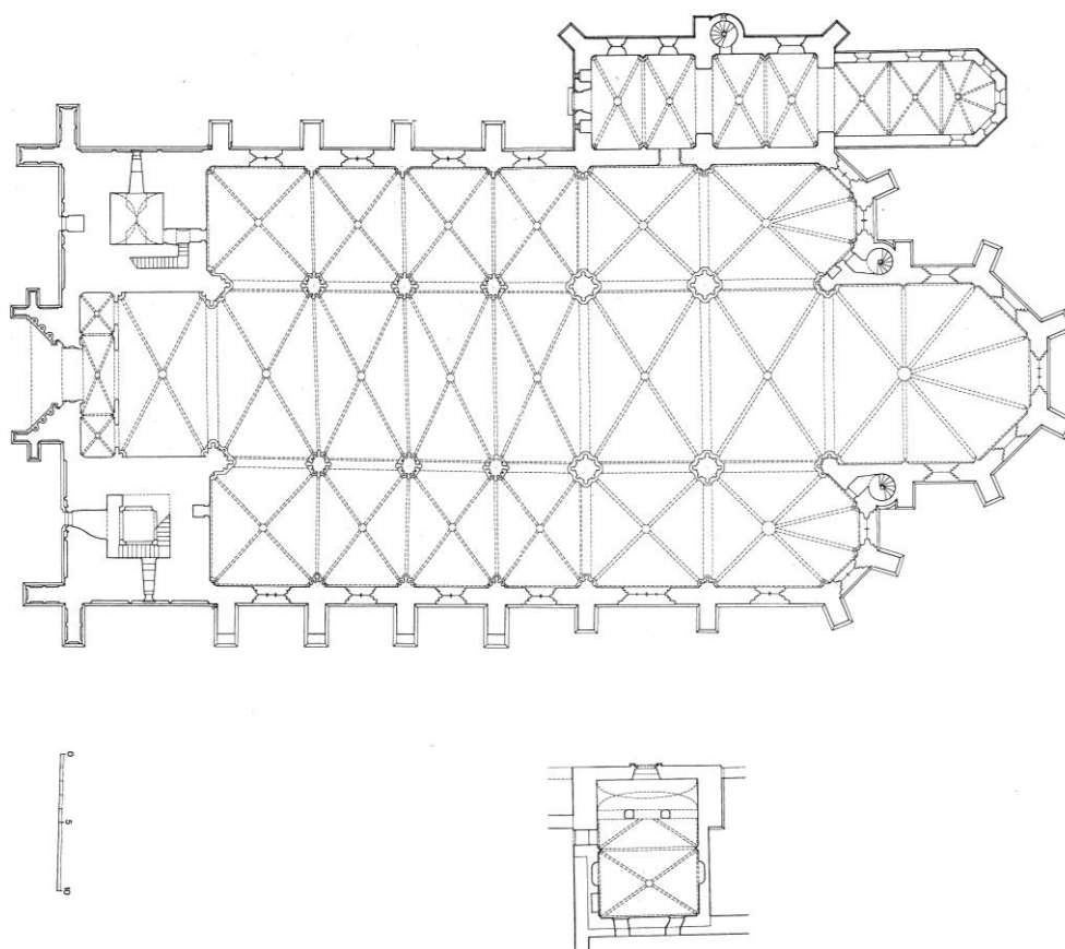
Zagreb, sačuvani dijelovi katedralnog sklopa: katedrala Uznesenja Blažene Djevice Marije, sakristija i biskupska kapela sv. Stjepana Prvomučenika tlocrt, postojeće stanje (Ivan Tenšek)
