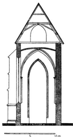
Lepoglava, crkva Bezgrešnog Začeca Blažene Djevice Marije, svetište poprečni presjek prema snimku M. Pilara (Horvat, Z. 1982, 8, sl. 4)
