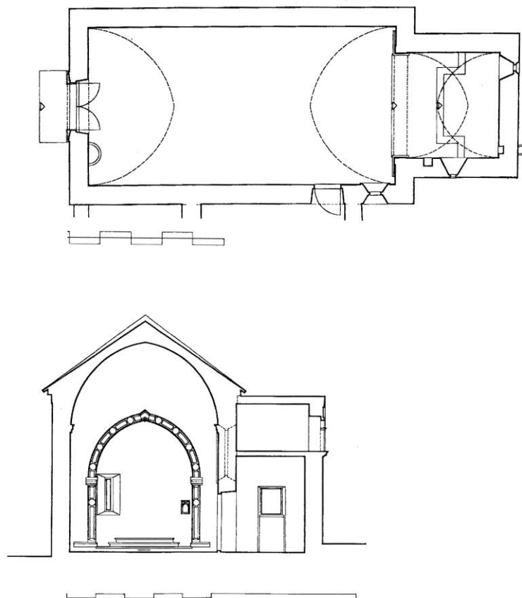
Rab., crkva sv. Frane „na groblju“, tlocrt (Domijan 2001, 205)
