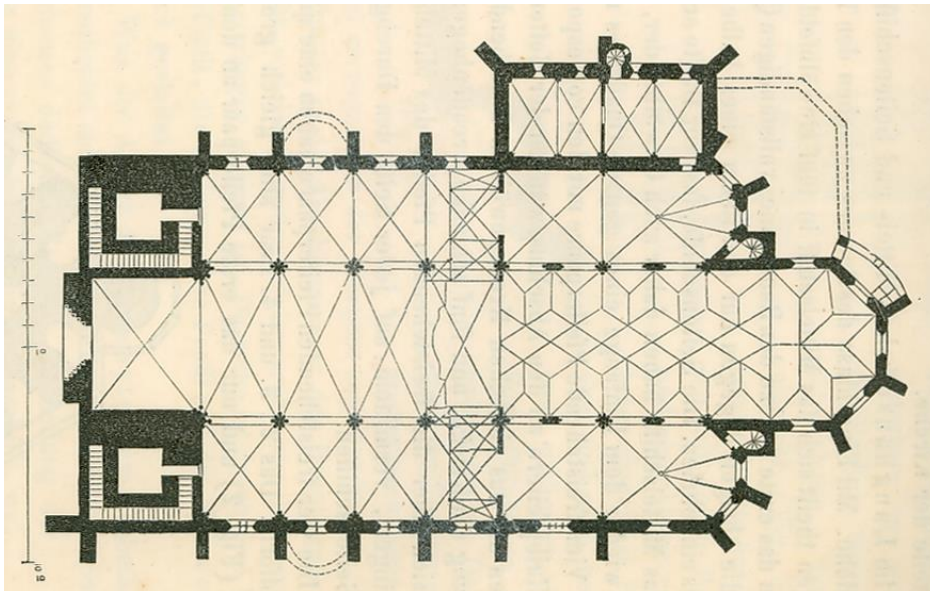
Tlocrt zagrebačke katedrale prije potresa (Weiss 1859)
