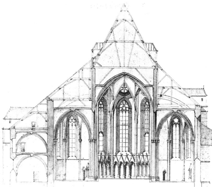
Zagrebačka katedrala prije regotizacije, poprečni presjek kroz svetište i sakristiju (snimak Schmit 1878.)
