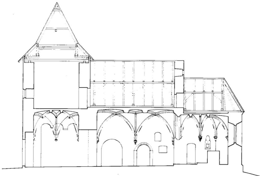
Belec, crkva sv. Jurja, uzdužni presjek (Vukičević-Samaržija 1993, 143)
