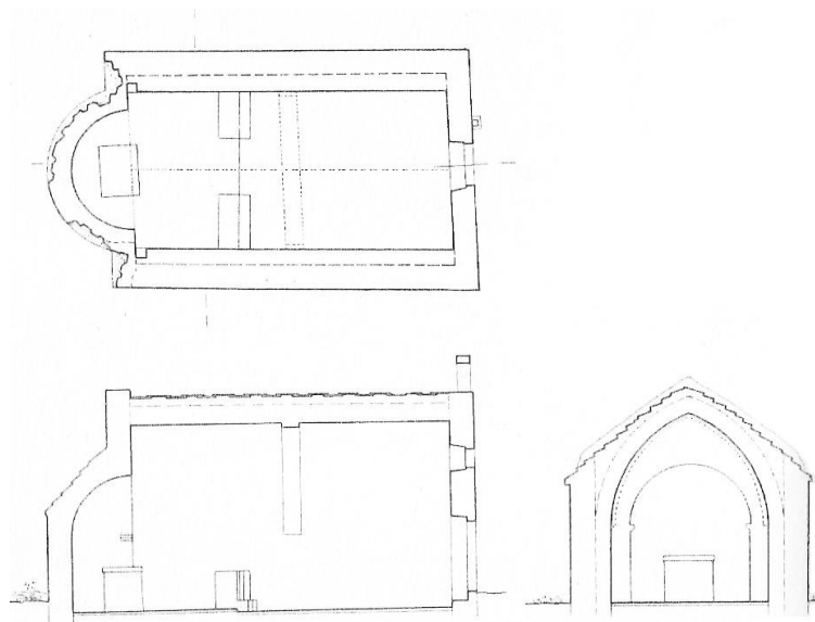
Sv. Juraj kod Jelovice, tlocrt i presjek (Mohorovičić 1958)
