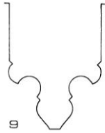
Požega, crkva sv. Lovre. Presjek rebara (Horvat, Z. 1992, 75)
