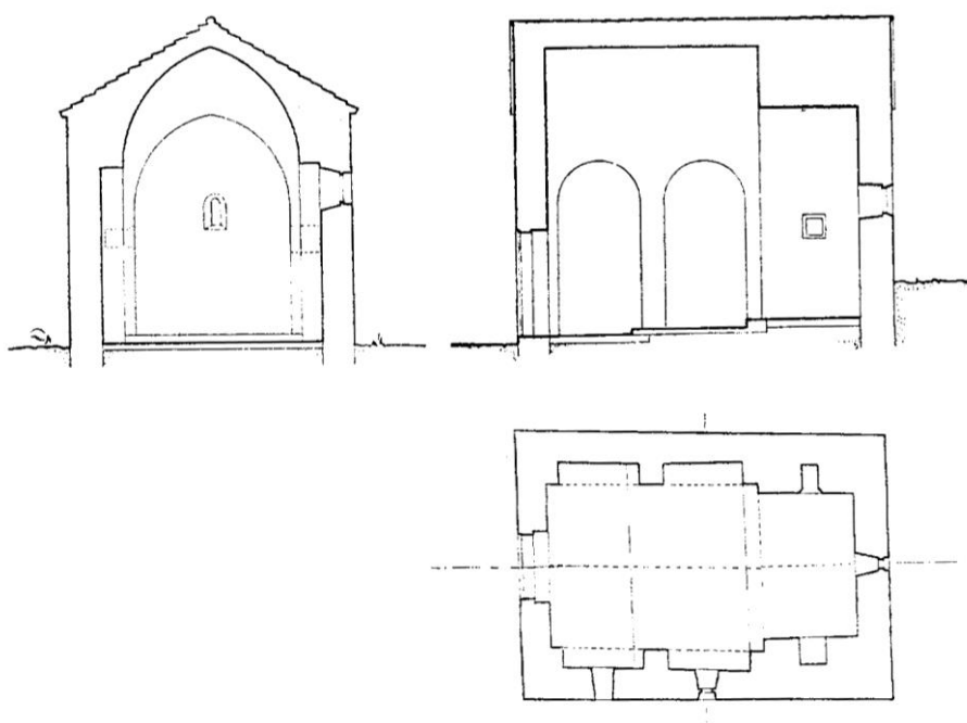
Žminj, Sv. Anton, tlocrt i presjeci (Mohorovičić 1958)
