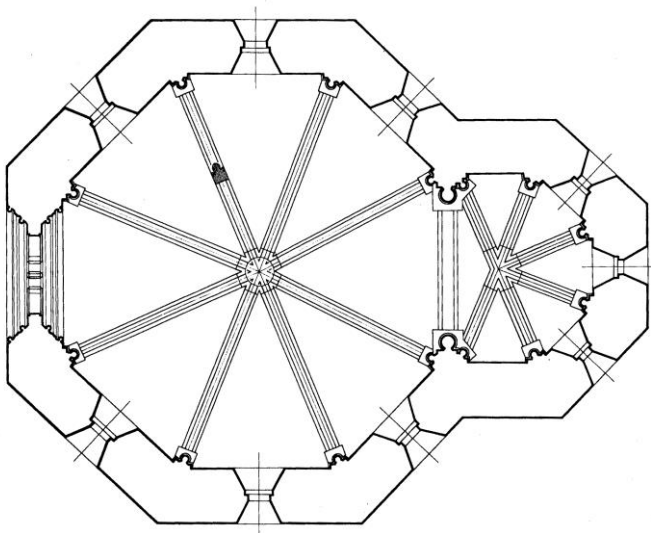
Medvedgrad, dvorska kapela, tlocrt, rekonstrukcija (Miletić - Valjato-Fabris 1987)
