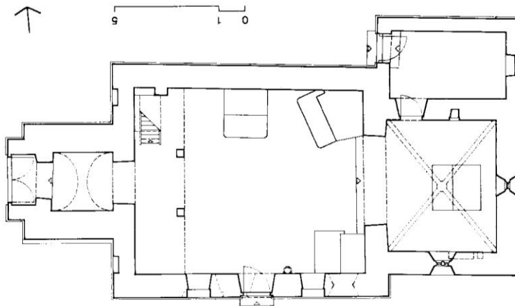
Martinščina, Sv. Martin, tlocrt (Vukičević-Samaržija, 1993. 176)
