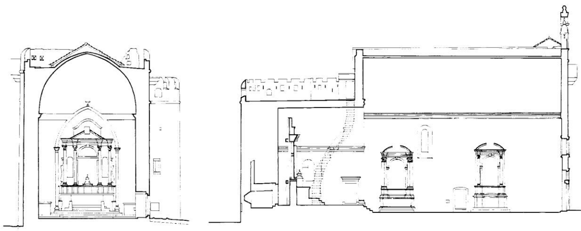
Vrboska, crkva sv. Marije od milosrđa, presjeci (Sekulić-Gvozdanović 1994, 49)
