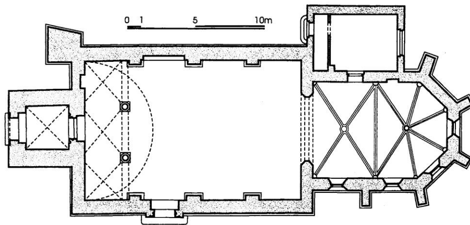
Križevci, crkva Sv. Križa, tlocrt (Balog, 2000, 18)
