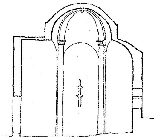
Sv. Krševan kod Glavotoka na Krku, presjek (prema: I. Petricioli)
