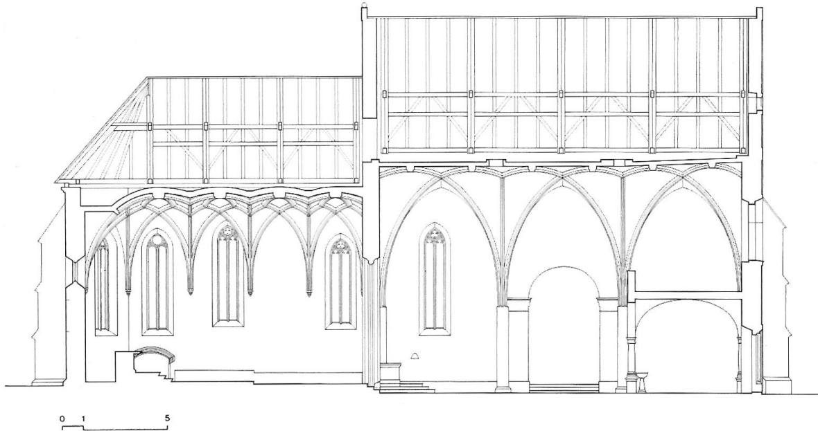
Remetinec, Sv. Marija, uzdužni presjek s pogledom na južni zid (Vukičević-Samaržija 1993, 197, sl. 191)
