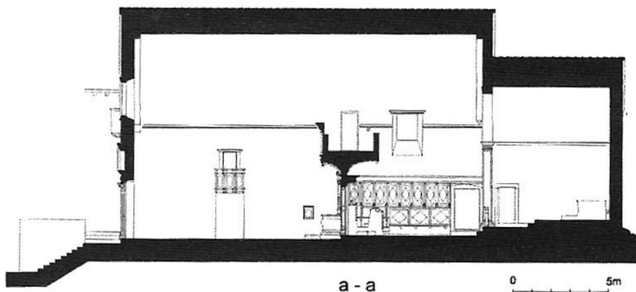
Hvar, franjevačka crkva Gospe od Milosti, presjek (Fisković 2010, 82)
