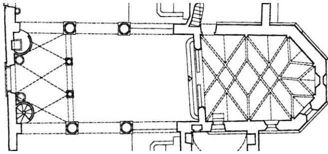
Roč, Sv. Bartol, tlocrt (Marković, V. 2004)
