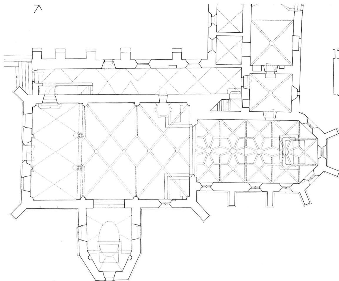
Remetinec, Sv. Marija, tlocrt crkve i dijela samostana (Vukičević-Samaržija 1993, 201, sl. 194)
