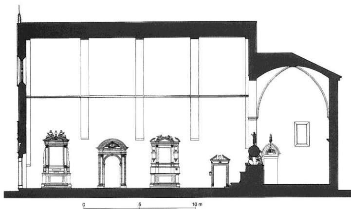
Badija - Otok kraj Korčule, franjevačka crkva, presjek (Fisković 2010, 91)
