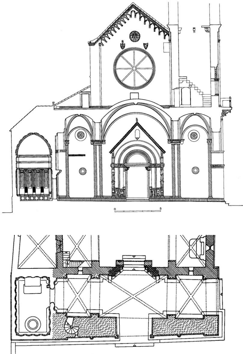
Predvorje trogirске katedrale, presjek i tlocrt (Stošić 1990)
