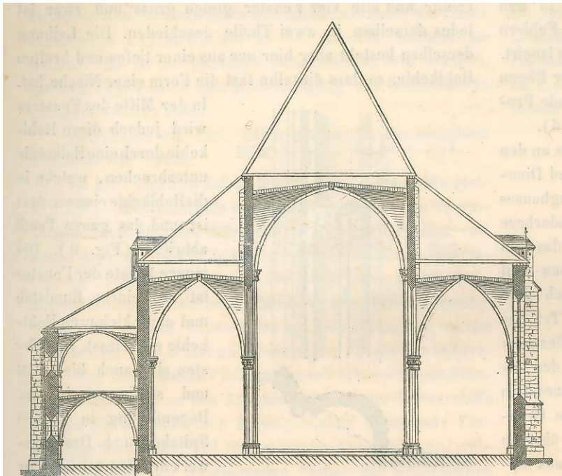
Zagreb, katedrala, poprečni presjek kroz svetište (Weiss 1859, 236, sl. 9)
