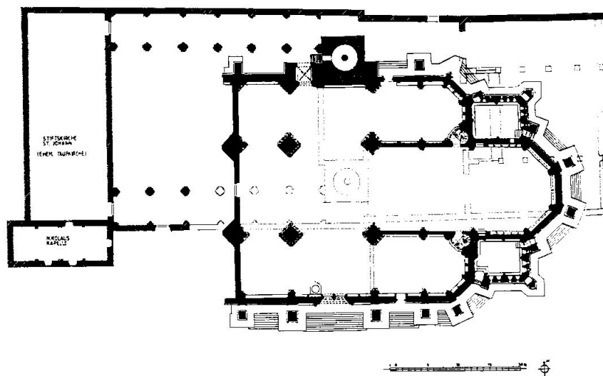
Katedrala u Regensburgu, prva gotička faza gradnje, tlocrt (Codreanu-Windauer & Schnieringer, 1990., 90)
