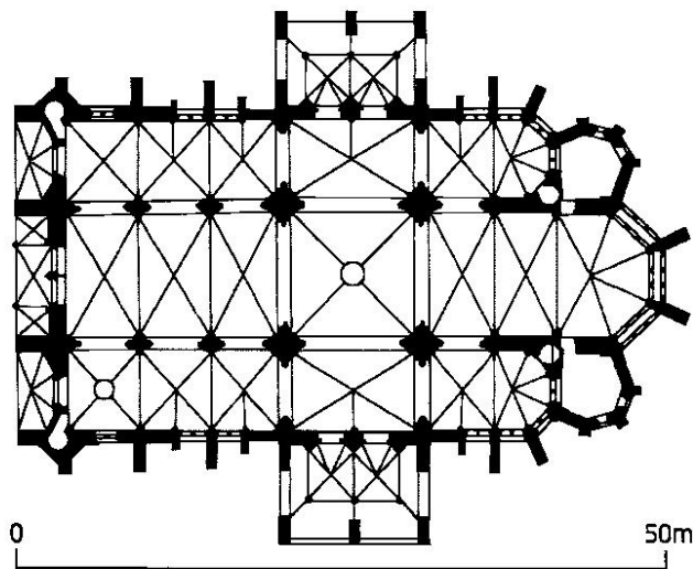
Troyes, zavjetna crkva Saint-Urbain, tlocrt (Schurr 2007, 182, sl. 195)
