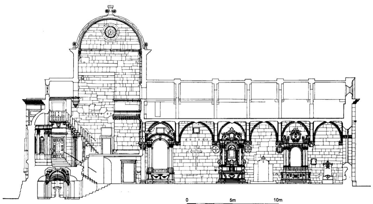
Šibenska katedrala, uzdužni presjek kroz južni bočni brod (Zavod za fotogrametriju) Radovi IPU, 3-6, 1982, 262, sl. 7
