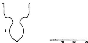
Topusko, cistercitska crkva, dijagonalno rebro glavnog broda (skica) (Horvat, Z. 1992, 74, sl. 80)
