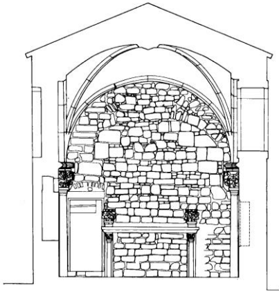
Split, kapela bl. Arnira, presjek s pogledom prema oltaru - Zavod za fotogrametriju, 1974. (Radovi IPU, 1982, 273)
