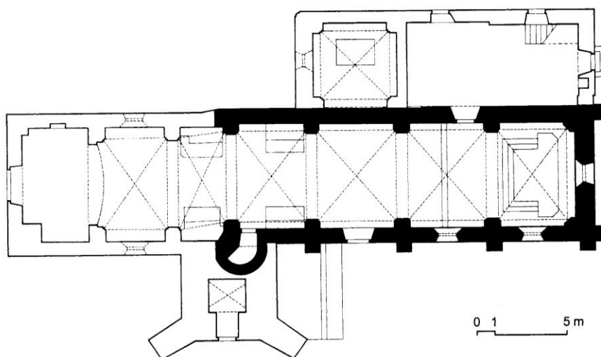
Gora, bivša templarska crkva Sv. Marije, tlocrt s istaknutim srednjovjekovnim dijelom (Vukičević-Samaržija 2001, 39, sl. 2)
