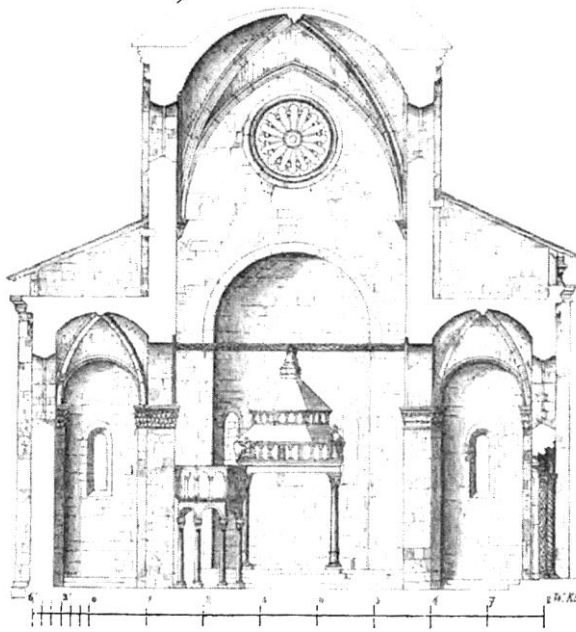
Trogirska katedrala, poprečni presjek (Eitelberger 1861: 206, sl. 48)
