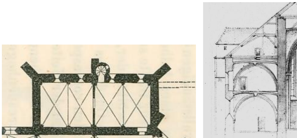
Zagrebačka katedrala, sakristija, stanje prije regotizacije, tlocrt (Weiss 1859)
