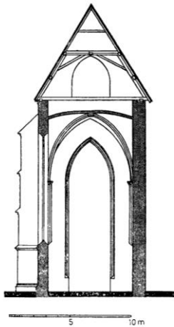
Lepoglava, crkva Bezgrešnog Začeca Blažene Djevice Marije, svetište poprečni presjek prema snimku M. Pilara (Horvat, Z. 1982, 8, sl. 4)
