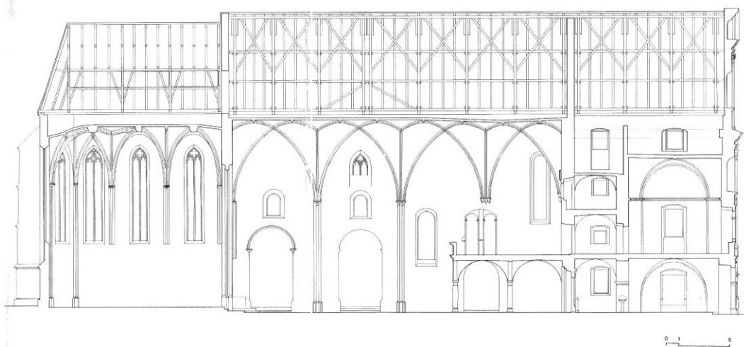
Lepoglava, crkva Bezgrešnog Začeca Blažene Djevice Marije, uzdužni presjek (Vukičević-Samaržija 1993, 168-169, sl. 163)
