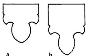
Rebra s bademastim zaključkom i zaliscima a. Čazma, crkva sv. Marije Magdalene b. Medvedgrad, kapela sv. Filipa i Jakova (Horvat, Z. 1992, 74, sl. 80a, b)
