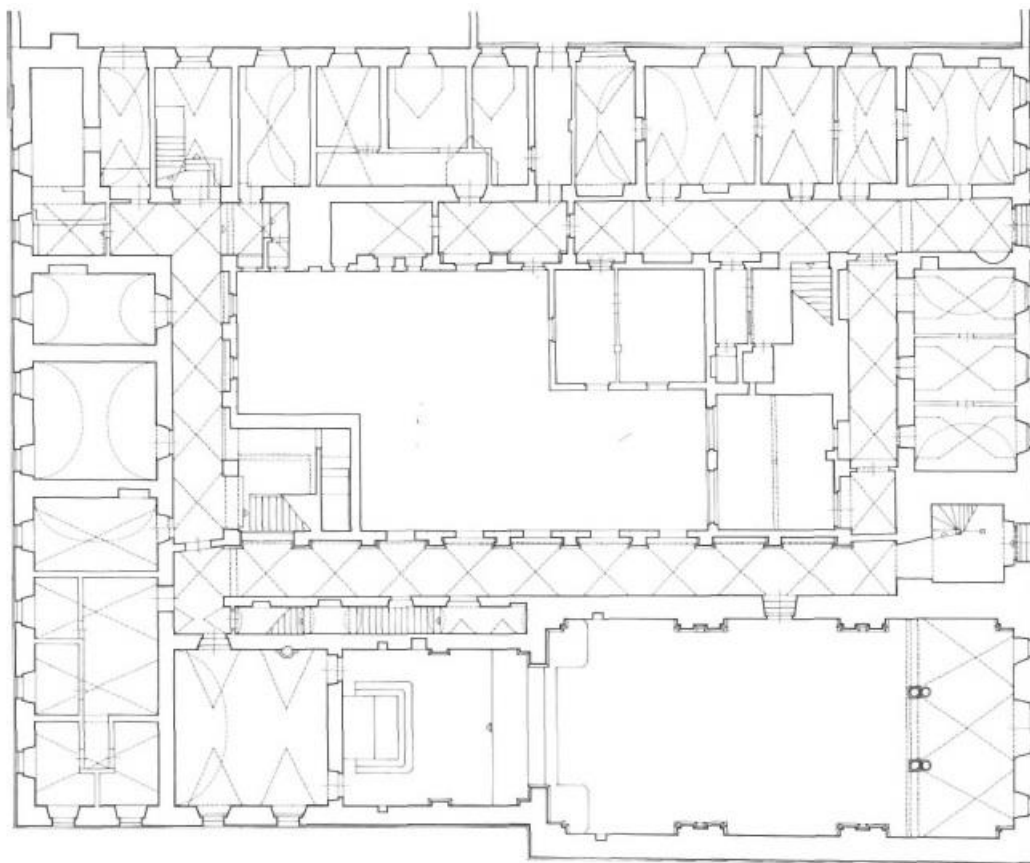
Sl. 8 – Tlocrt prizemlja samostana i crkve sv. Ane (izvor: Đurđica Cvitanović, Pavlinski samostan i crkva sv. Ane , u: Žarko Domljan (ur.), Križevci – grad i okolica , str. 160)
