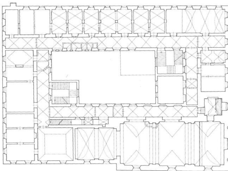
Sl. 9 – Tlocrt kata samostana i crkve sv. Ane (izvor: Đurđica Cvitanović, Pavlinski samostan i crkva sv. Ane , u: Žarko Domljan (ur.), Križevci – grad i okolica , str. 161)
