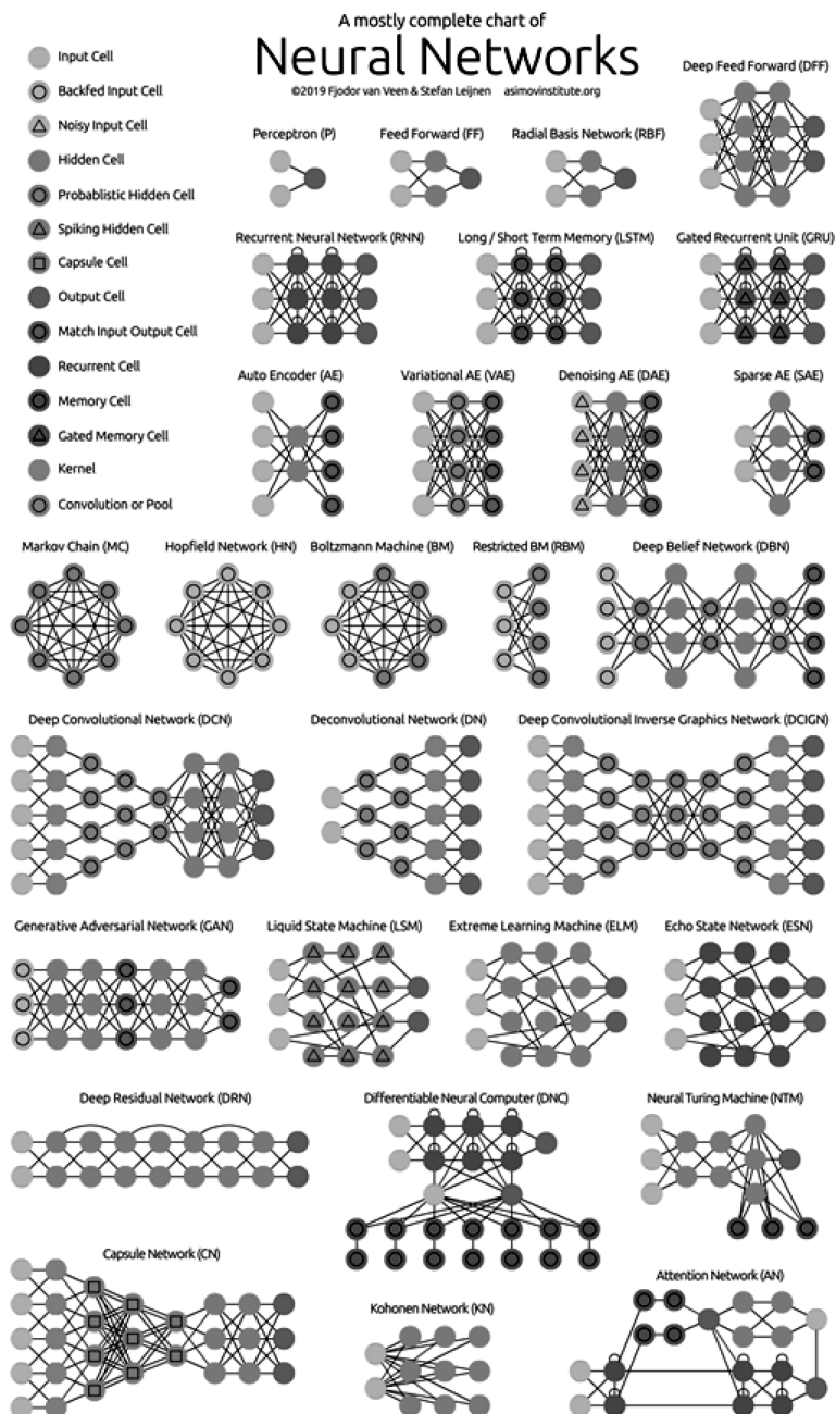
Slika 1. Gotovo potpuni prikaz neuronskih mreža (Preuzeto iz Van Veen i Leijnen 2020).
