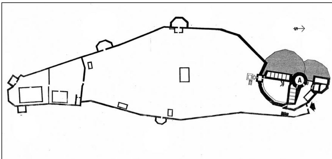
prilog 47 - tlocrt utvrde Ostrožac - A – pozicija prvobitne branič-kule (prema Truhelka, Naši gradovi , str. 23. izradio Zorislav Horvat)
