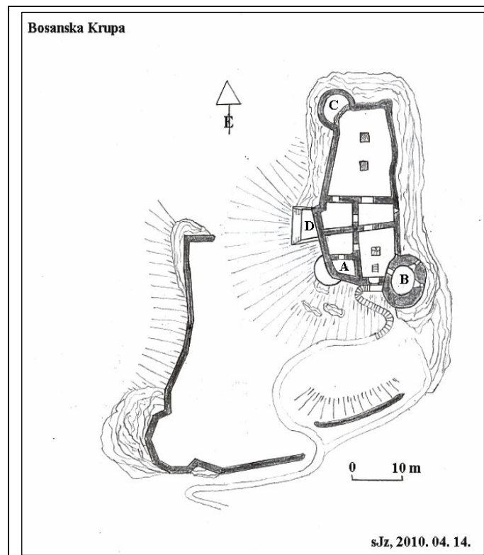
prilog 42 - tlocrt Krupa na Uni ( http://jupiter.elte.hu/terkep+lista2.php )
