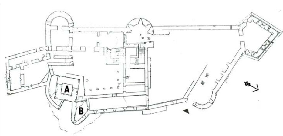
prilog 60 - tlocrt utvrde Samobor
