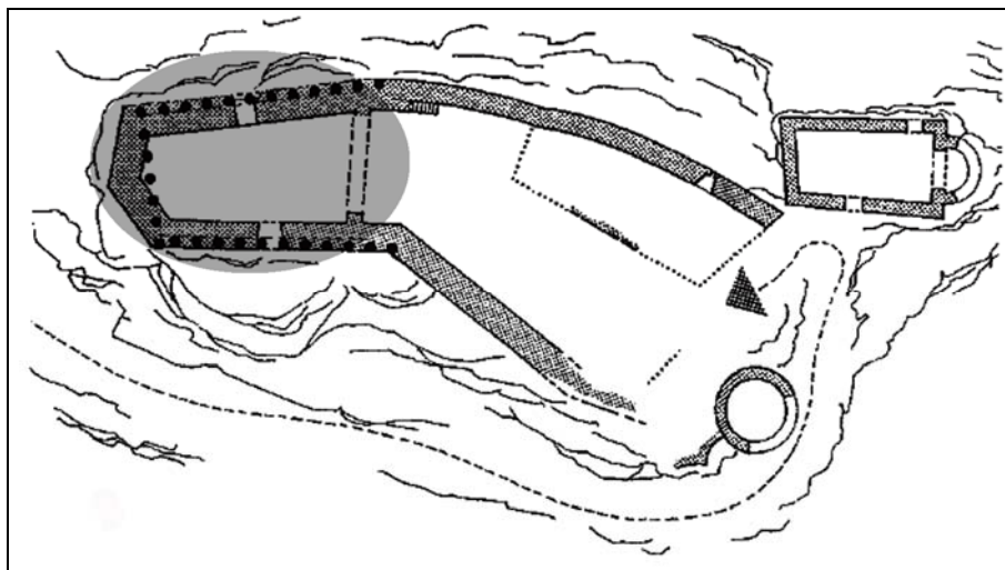
prilog 58 - tlocrt utvrde Okić - u crvenom krugu - položaj prvobitne branič kule iz sredine 13. stoljeća (Horvat, „Stilska stratigrafija burgova“, str. 45.)
