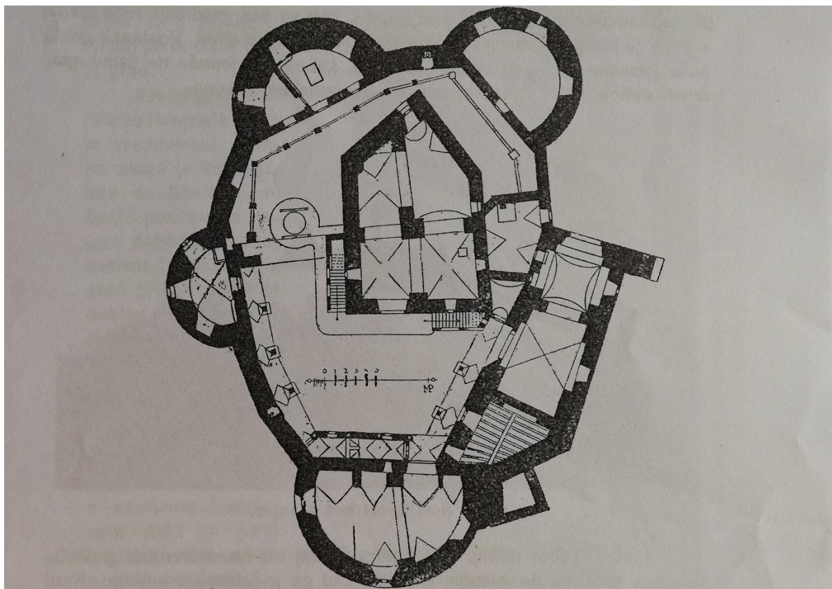
Slika 8. Tlocrt prizemlja V. Tabora (Szabo 2006, 77)
