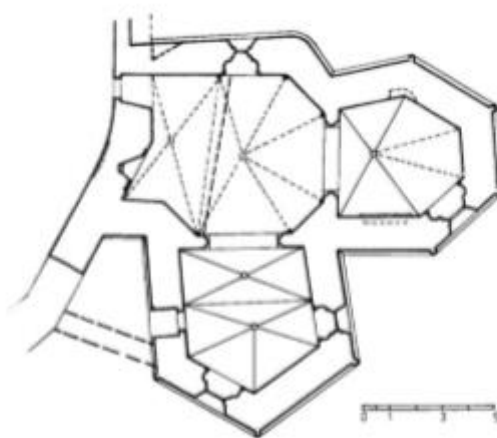
Slika 7. Tlocrt dvorske kapele Presvetog Trojstva u Brinju (Horvat 1958, 53)
