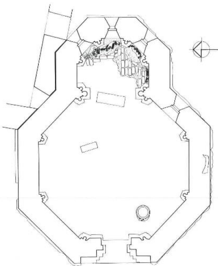
Slika 6. Tlocrt kapele sv. Filipa i Jakova (Miletić – Valjato-Fabris 2003, 16)
