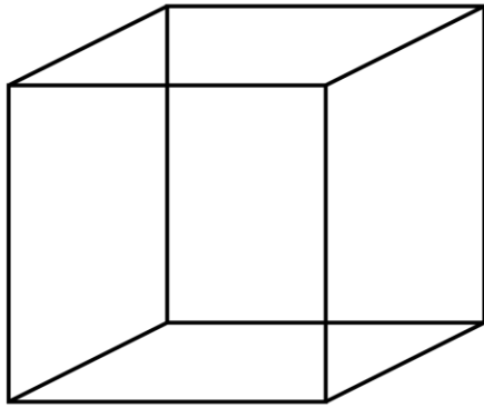
Slika 4. Neckerova kocka
