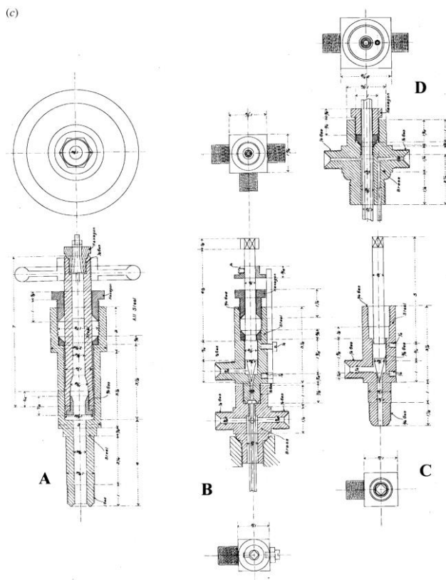
Slika 1 - Wittgensteinovi nacrti propelera sa malim mlaznim motorima na krajevima njegovih krakova
