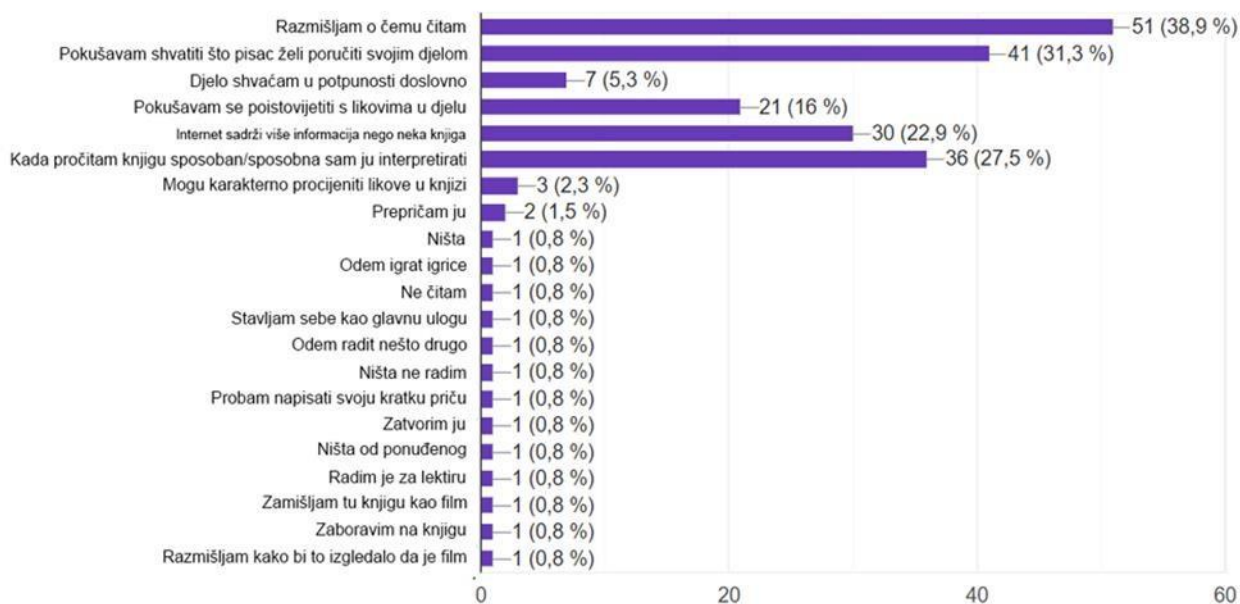
Slika 8: Bit čitanja
