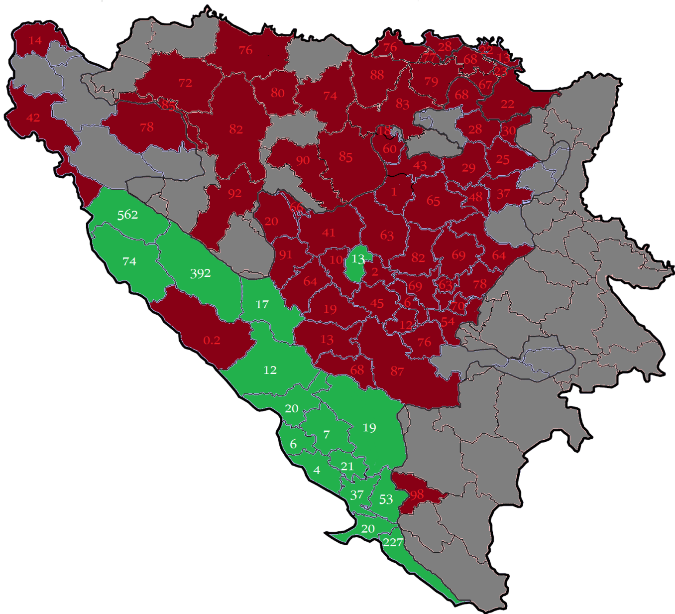
Slika 1: Promjena broja Hrvata između dvaju zadnjih popisa stanovništva na područjima gdje čine značajniji udjel u stanovništvu. Na zelenim područjima se povećao broj Hrvata, dok se na crvenim područjima smanjio. Brojevi označavaju postotke. 33
